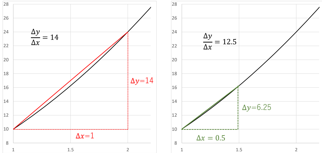
図1 微分の考え方（理論値:黒線と点線で囲まれた面積 ⇒ 近似値:赤（緑）線と点線で囲まれた三角形の面積）
