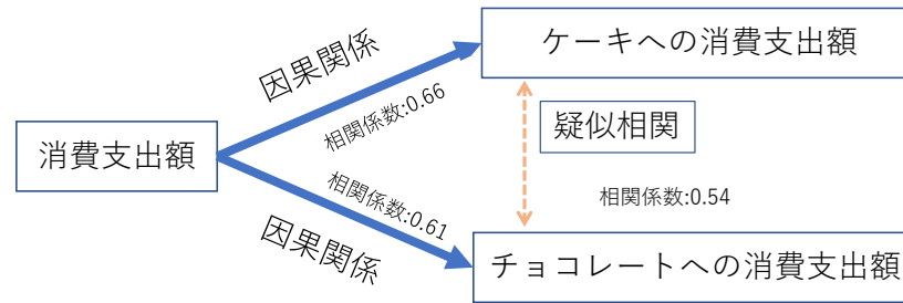
図 14 疑似相関
