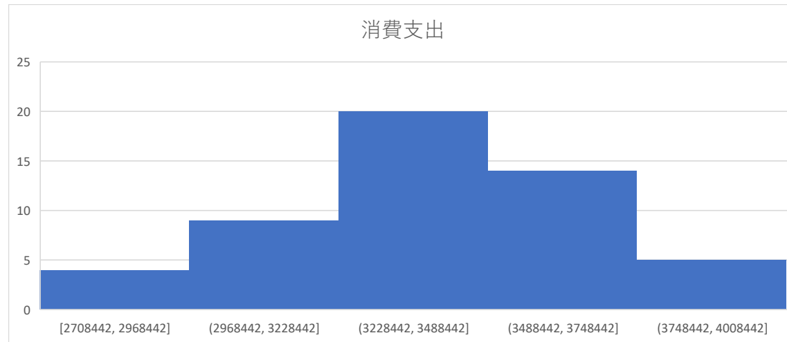
図7 消費支出のヒストグラム
