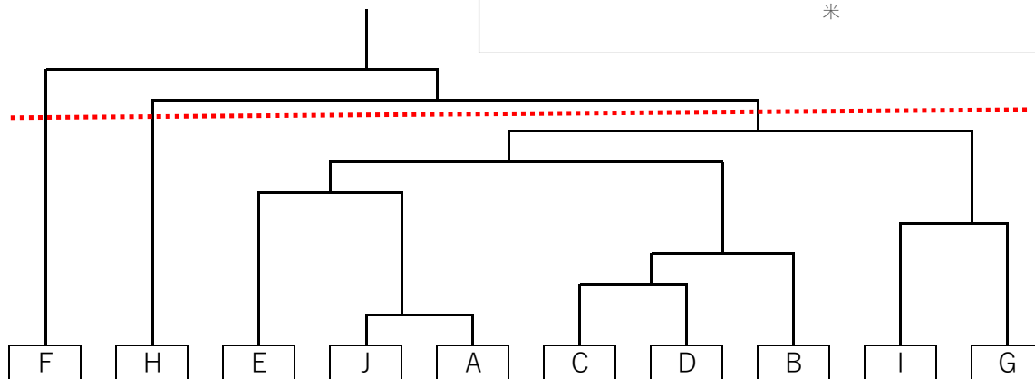
図 19 例題のデンドログラム (樹形図)
