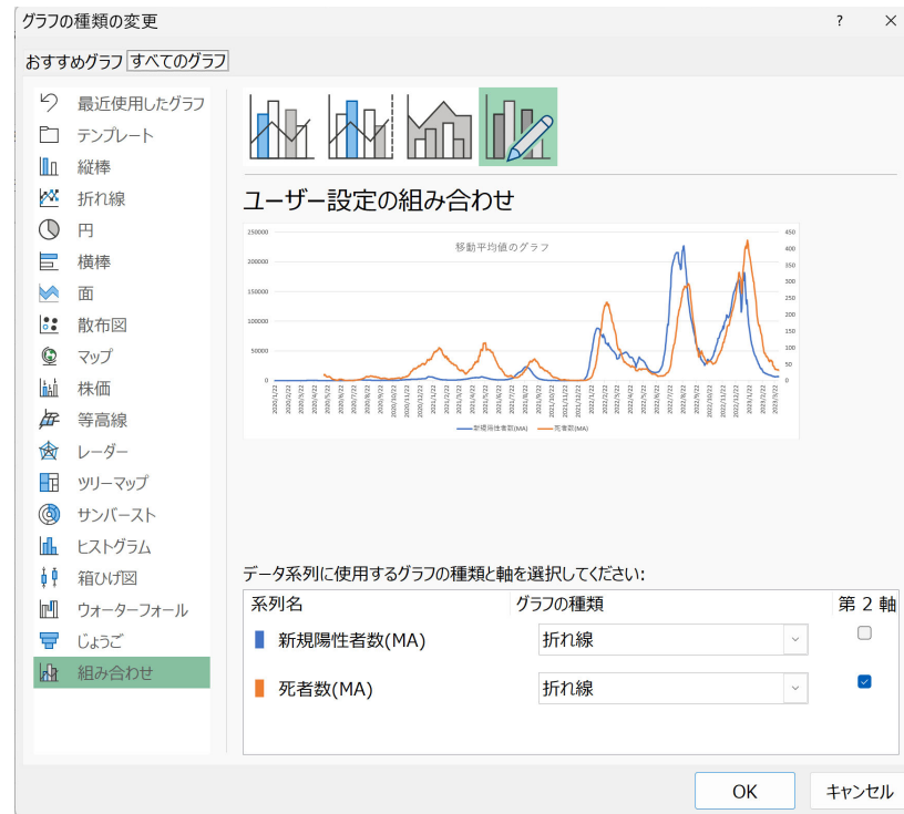
図 23 原系列の 2 軸グラフの設定
