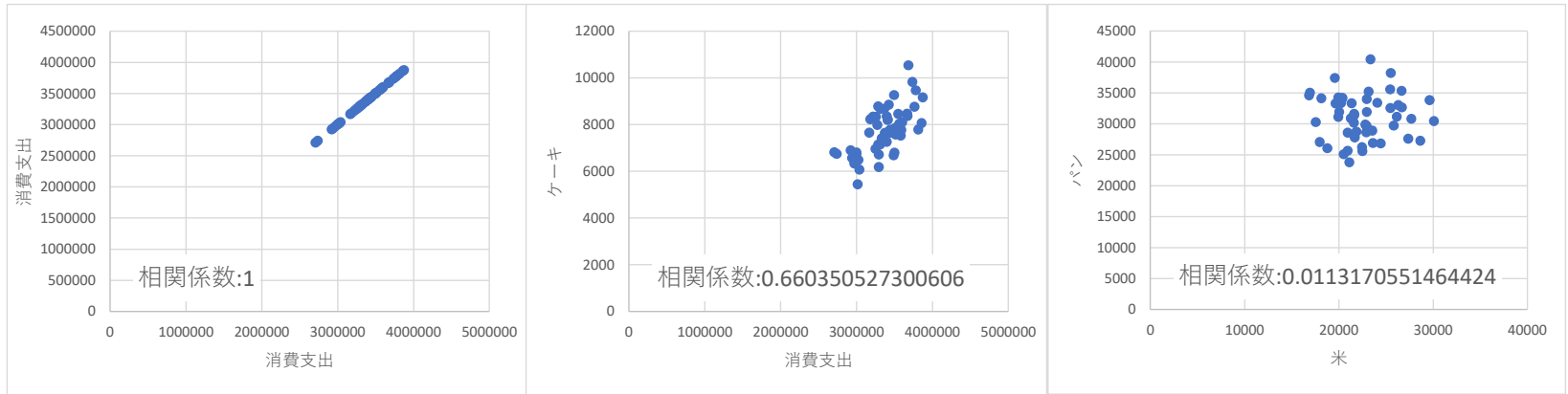
図9 3つの散布図と相関係数
