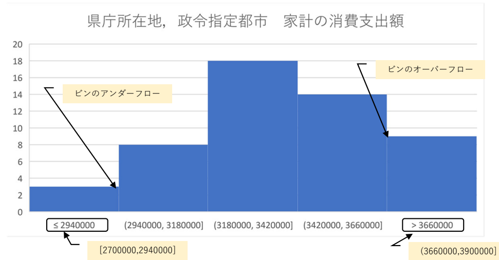
図 35 きりの良い階級のヒストグラム
