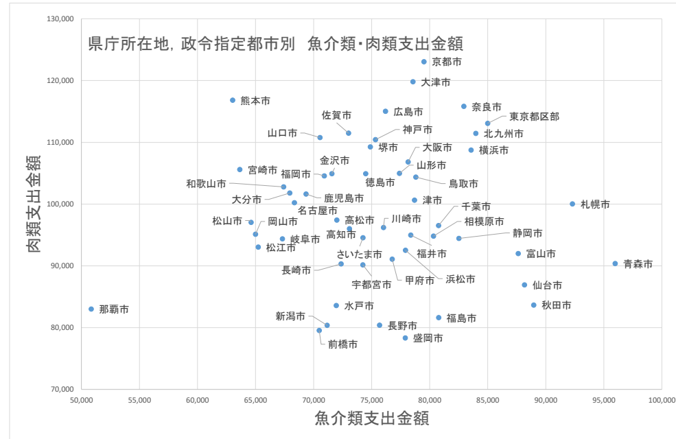
図 15 散布図の例
